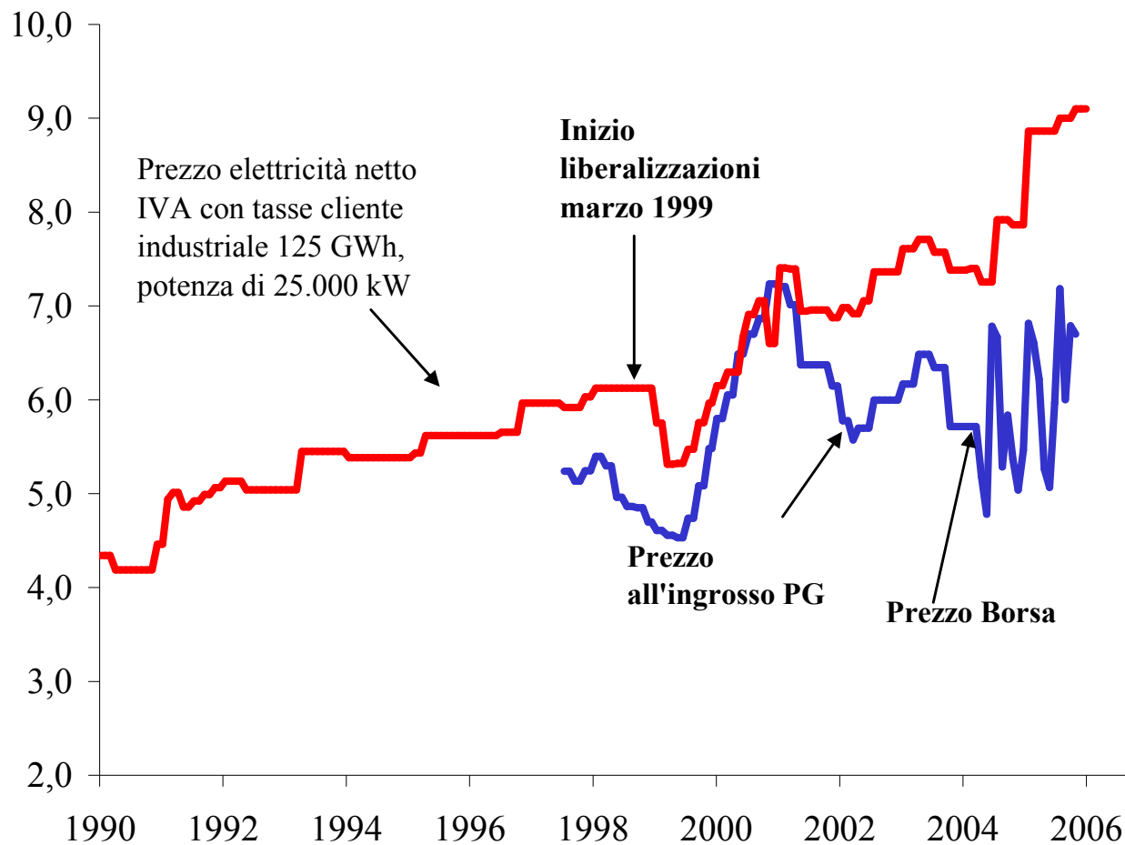
Fig. 7: Tariffe e prezzi all'industria e prezzi all'ingrosso (cents/kWh)
